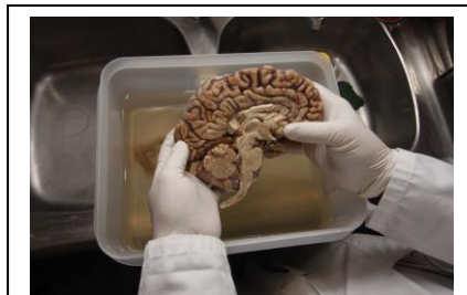
La superficie interna del cerebro humano revela su patrón básico de organización.
