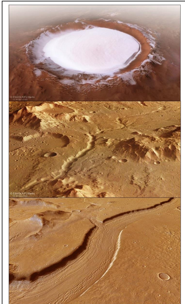
Tres imágenes de Marte tomadas por la misión europea Mars Express donde la presencia de agua presente o pasada es evidente. Imagen superior: Cráter Korolev cubierto de agua helada. Imágenes del medio e inferior: surcos de antiguos ríos de agua líquida. Imágenes de ESA/DLR/FU Berlin.
