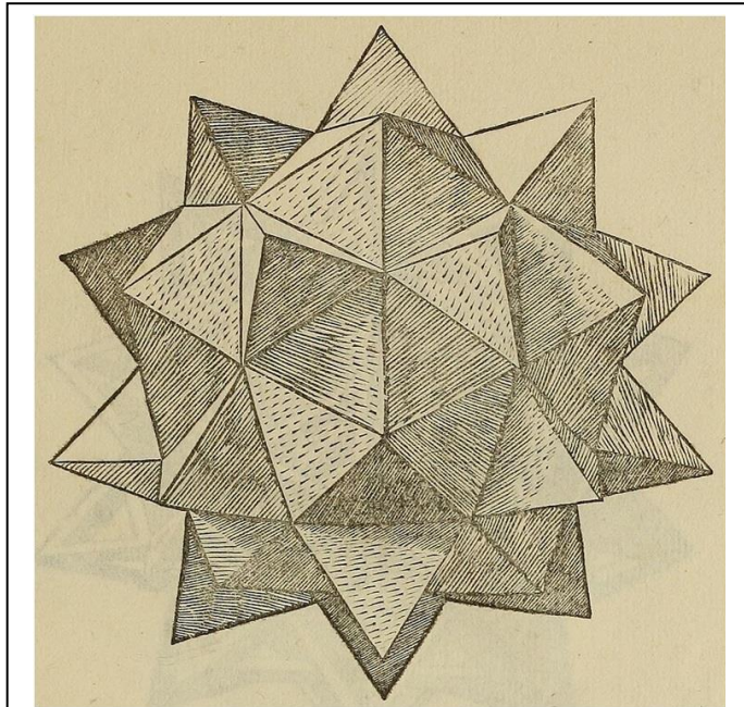
Fig. 3. Poliedro estrellado.
