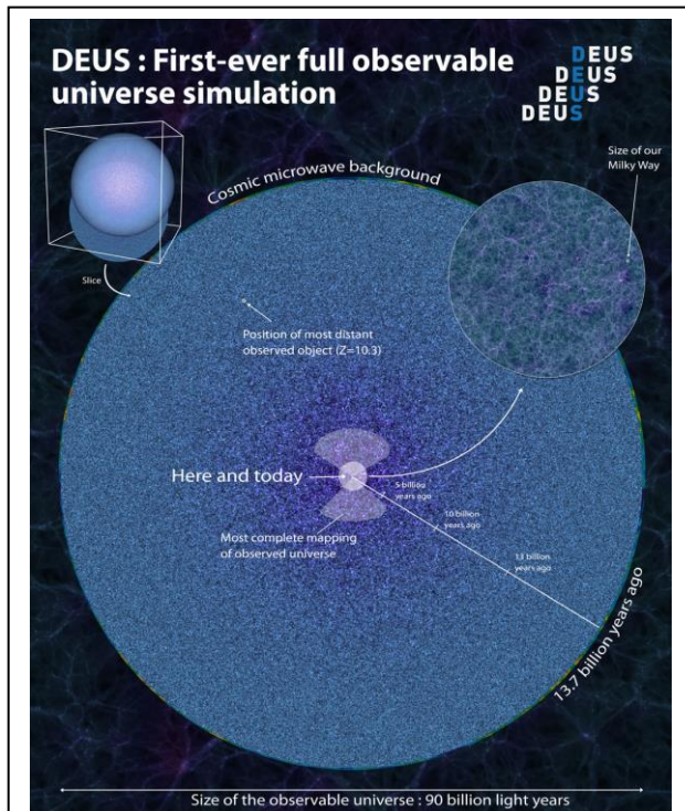
Representación gráfica del concepto actual de Universo observable: una hipersfera de 3 dimensiones espaciales, con un radio de ~45.000 millones de años luz, y una dimensión temporal con un radio de 13.800 millones de años. El observador se encuentra en el centro de la hipersfera, cuya superficie se expande de manera continua. Cortesía del Consorcio DEUS.
