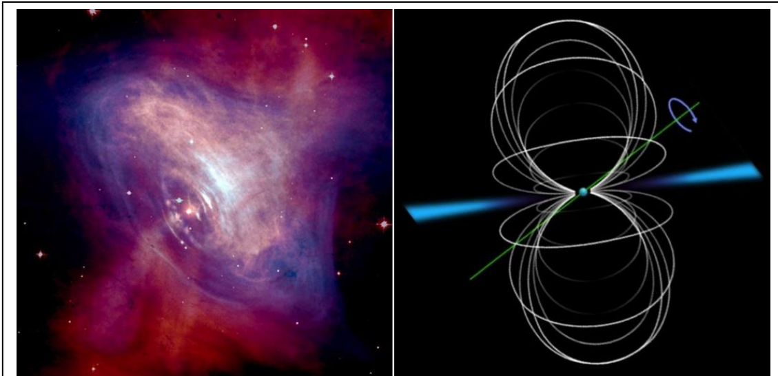
Izquierda: imagen óptica y de rayos X de la estrella de neutrones y el viento de púlsar circundante (con chorros en la dirección del eje de rotación) situados en el centro de la Nebulosa del Cangrejo, formada por los restos de la supernova que dio lugar a la estrella de neutrones y que fue observada en la Tierra en 1540 d.C. (Licencia: dominio público. Autoría: NASA/HST/ASU/J. Hester et al.). Derecha: esquema de una estrella de neutrones (esfera central) que muestra las líneas de campo magnético (en blanco), el eje de giro (en verde) y los haces de radiación electromagnética emitidos desde los polos magnéticos (en azul). (Licencia: CC BY-SA 3.0. Autoría: User:Mysid - Wikimedia Commons).
