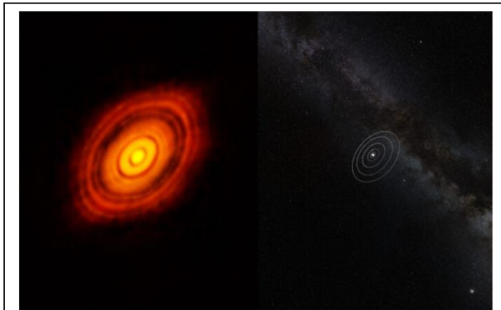
A la izquierda, disco protoplanetario alrededor de la estrella HL Tauri, utilizando imágenes de los telescopios ALMA y Hubble. A la derecha, montaje para comparar el tamaño del Sistema Solar con HL Tauri. Créditos: ALMA (ESO/NAOJ/NRAO)
