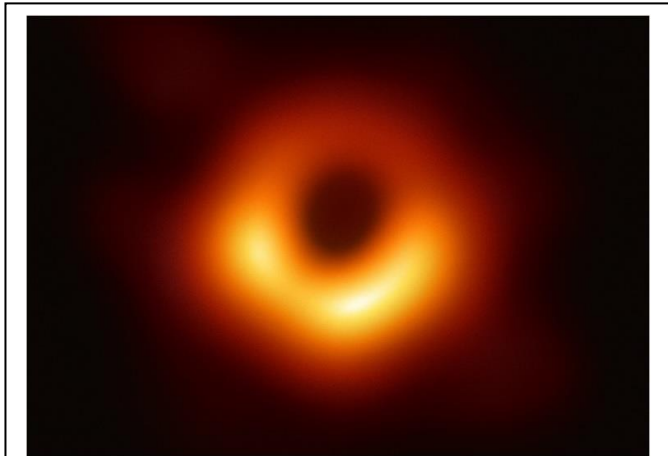
La primera fotografía de un agujero negro, publicada en abril de 2019.
