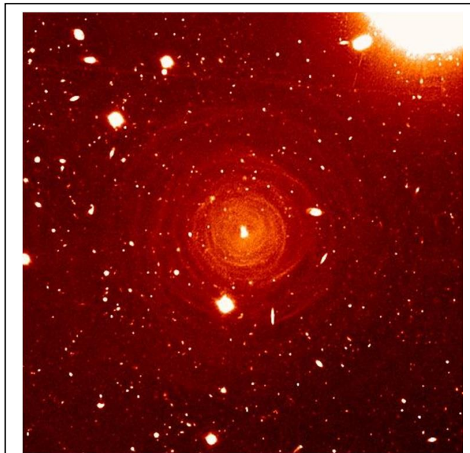
Imagen de la emisión del polvo de la envoltura circunestelar IRC+10216.
