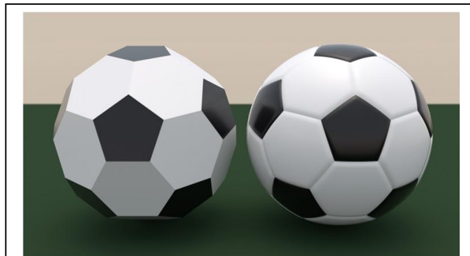
Fig. 4. Icosaedro truncado
